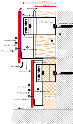
VERTIKALNI PRESJEK (2) SPOJ VENTILIRANOG SOKLA I VENTILIRANE FASADE
