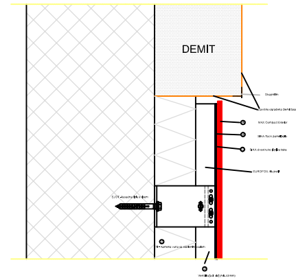
VERTIKALNI PRESJEK (7) SPOJ SA DEMIT FASADOM
