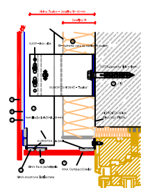
VERTIKALNI PRESJEK (5) SPOJ SA BRAVARIJOM - PODGLED
