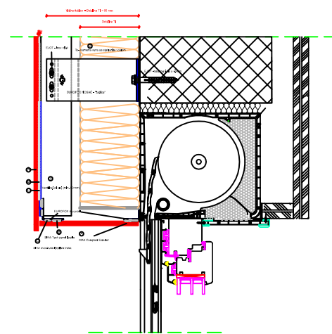
VERTIKALNI PRESJEK (6) SPOJ SA KUTIJOM ROLETA - PODGLED
