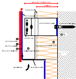
VERTIKALNI PRESJEK (1) SPOJ SOKLA (DEMIT, TERAPLAST...) I VENTILIRANE FASADE
