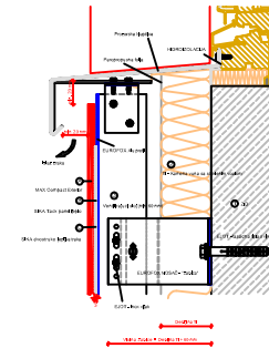
VERTIKALNI PRESJEK (3) SPOJ VENTILIRANE FASADE I PROZORSKE KLUPČICE
