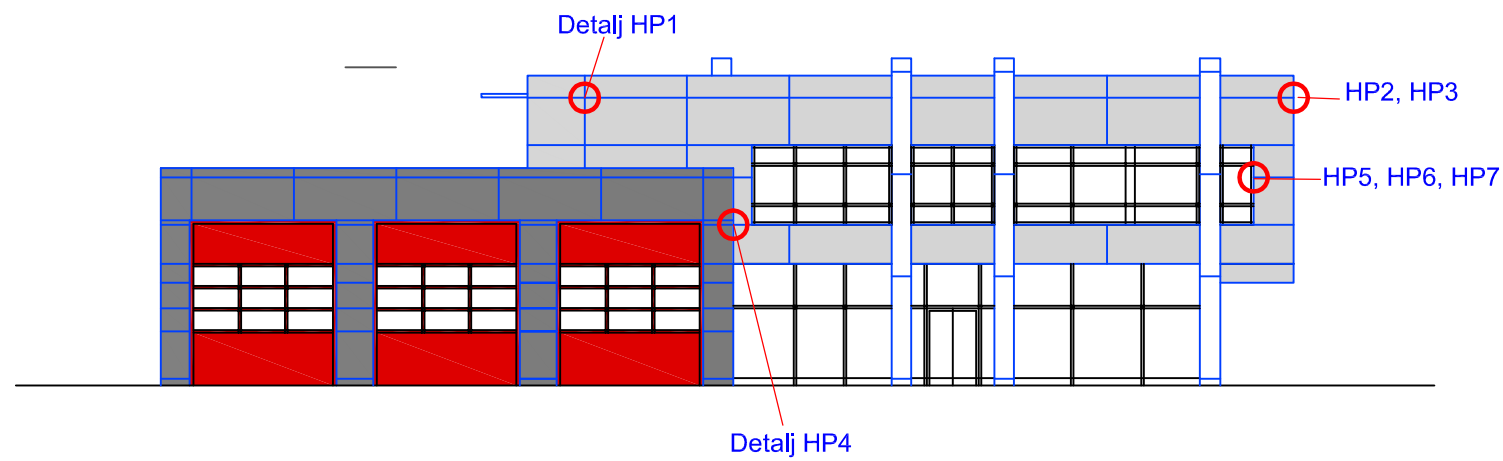
PROČELJE 1
