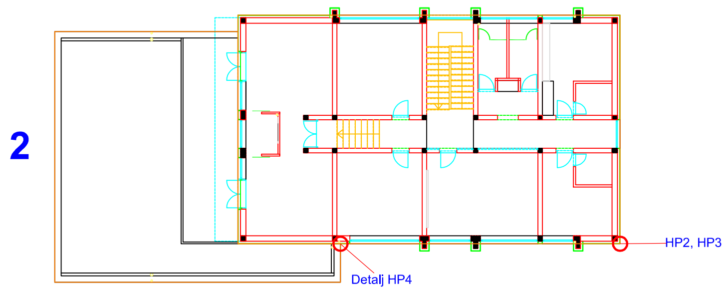
TLOCRT
