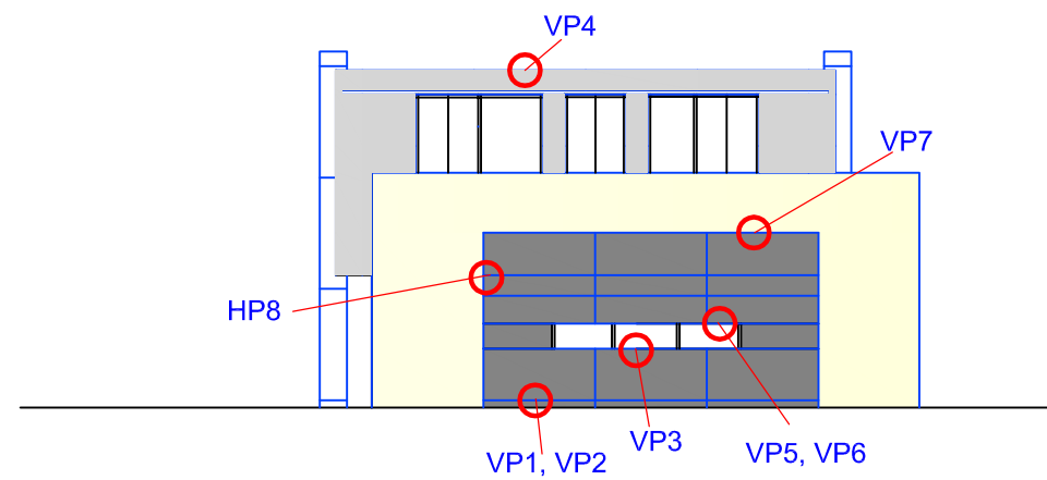
PROČELJE 2
