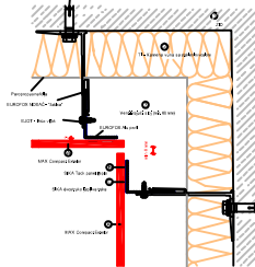
HORIZONTALNI PRESJEK (4) UNUTARNJI KUT
