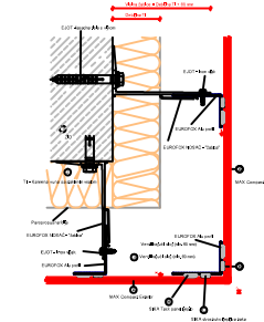
HORIZONTALNI PRESJEK (3) KUTNI SPOJ - "GERUNG"
