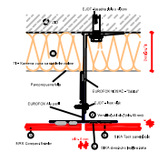
HORIZONTALNI PRESJEK (1) SPOJ PLOČA NA "T" PROFILU
