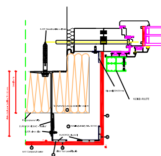
HORIZONTALNI PRESJEK (7) ŠPALETA, SPOJ SA BRAVARLIJOM I VODLICAMA ZA ROLETE
