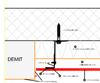
HORIZONTALNI PRESJEK (8) SPOJ SA DEMIT FASADOM
