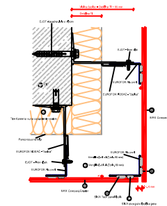
HORIZONTALNI PRESJEK (2) KUTNI SPOJ
