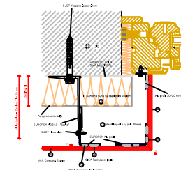
HORIZONTALNI PRESJEK (6) ŠPALETA, SPOJ SA BRAVARLIJOM - "GERUNG"
