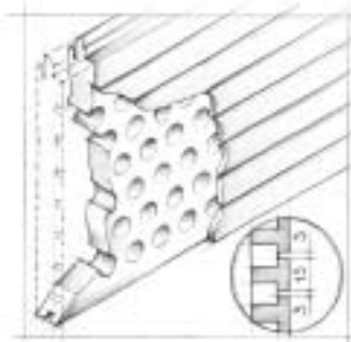
Tipologia 13/3 Perforazione 12% Type 13/3 12% drilling
