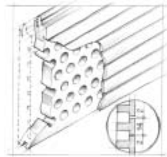
Tipologia 14/2 Perforazione 7% Type 14/2 7% drilling
